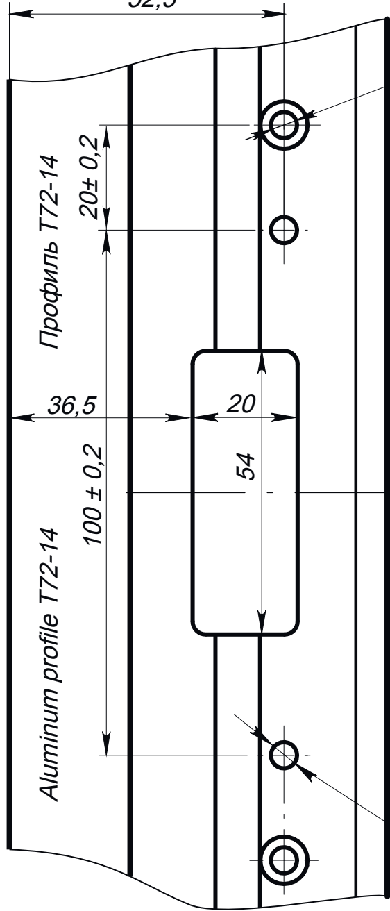
Вид Б-Б View Б-Б
