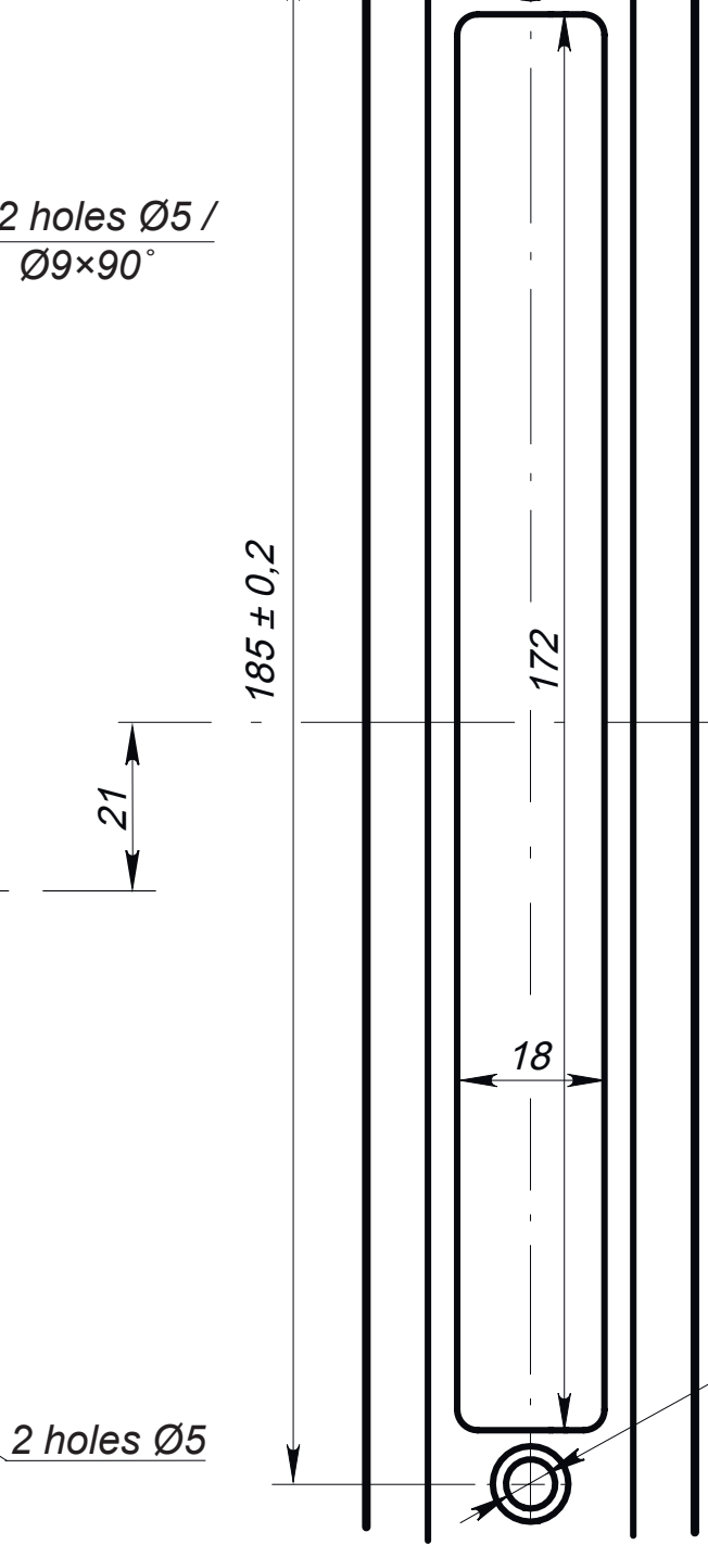
Вид А-А View А-А
