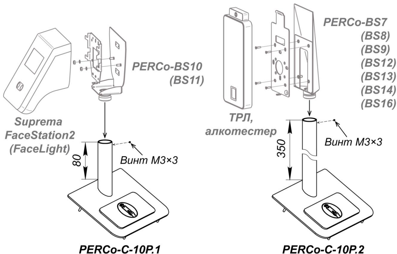
Рисунок 30. Внешний вид боковых крышек PERCo-C-10P.1 , PERCo-C-10P.2
