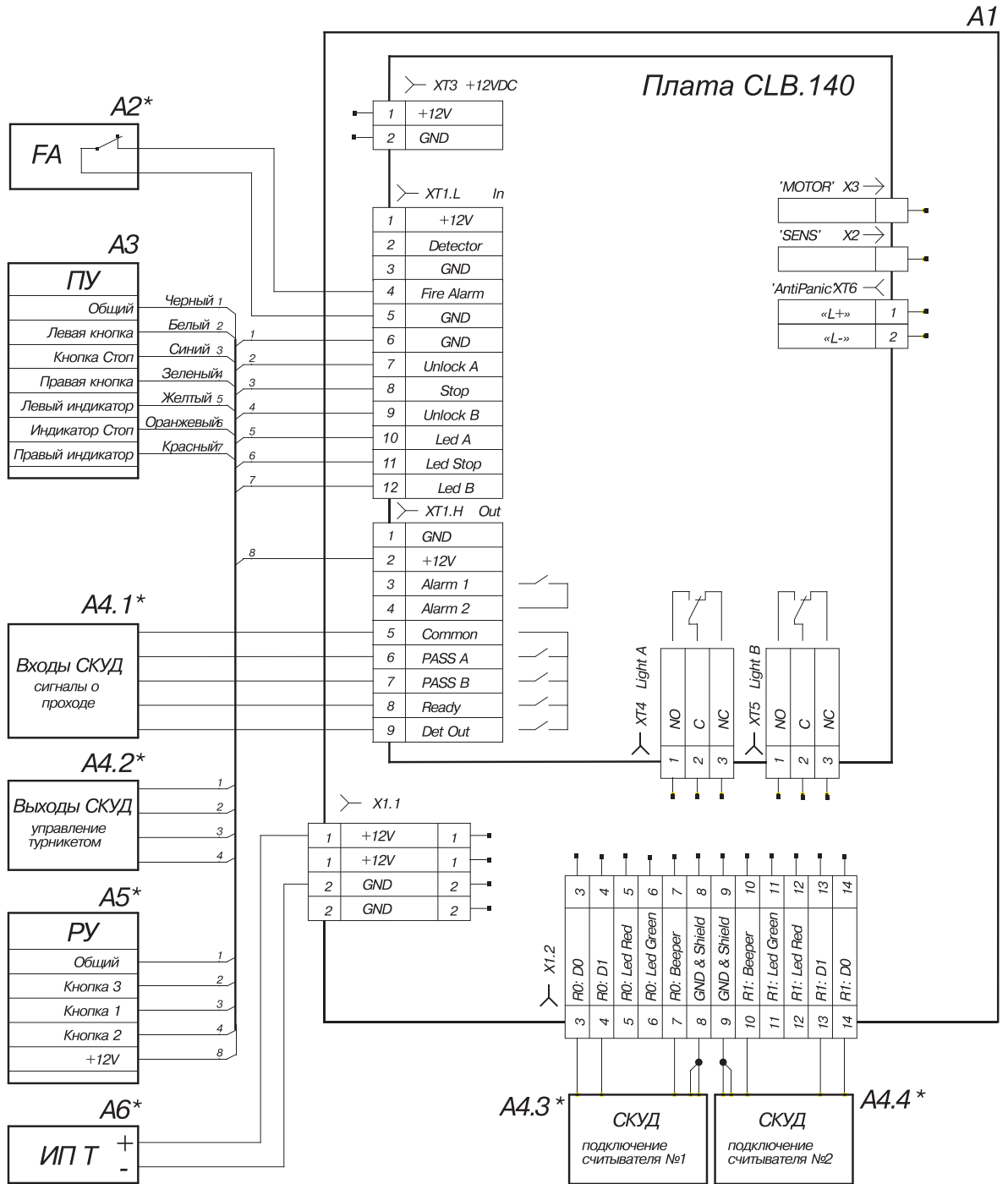
Схема соединений турникета PERCO-TV01.9А и дополнительного оборудования
