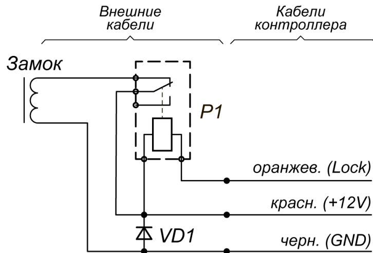
P1 - промежуточное реле, 12V / 10A
